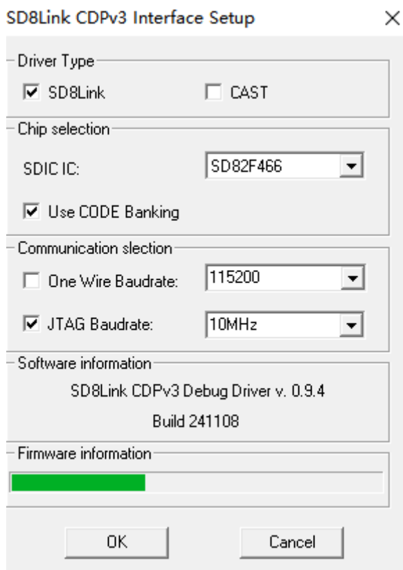
图 2.4.3 更新进度条
