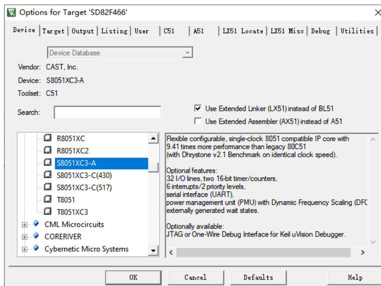
图 5.3 链接器 LX51
