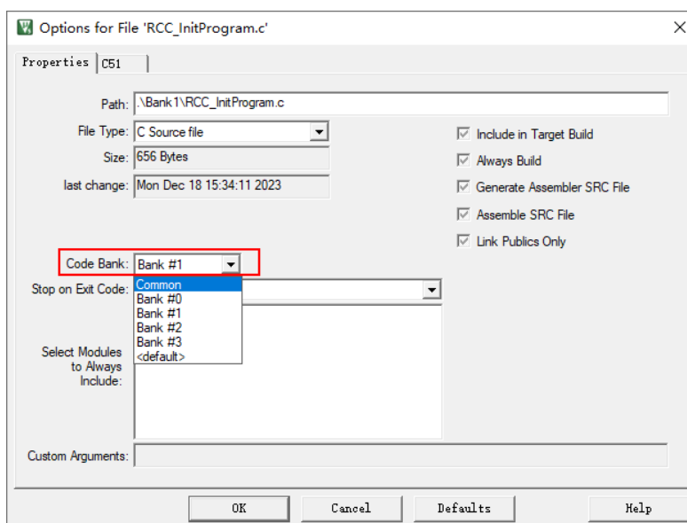
图 5.6.2 文件设置
