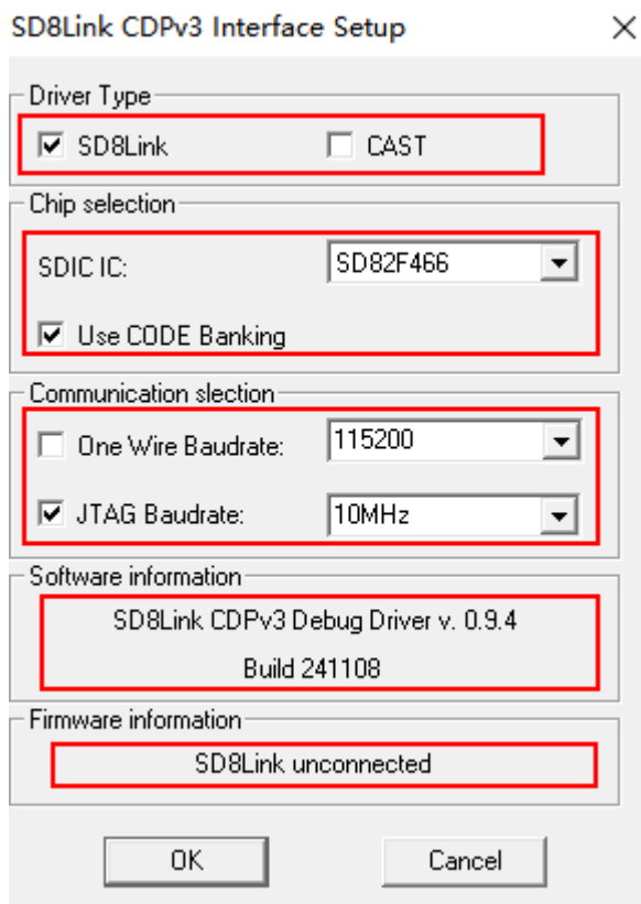
图 2.4.1 驱动设置
