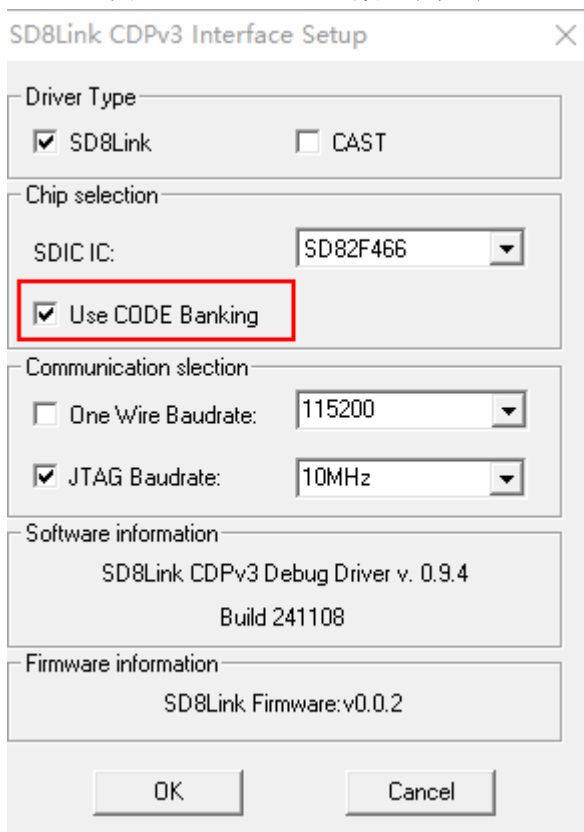
图 5. 4. 2 调试器设置
